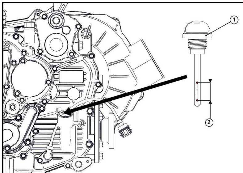
① Olejová měrka ② Doporučený rozsah
